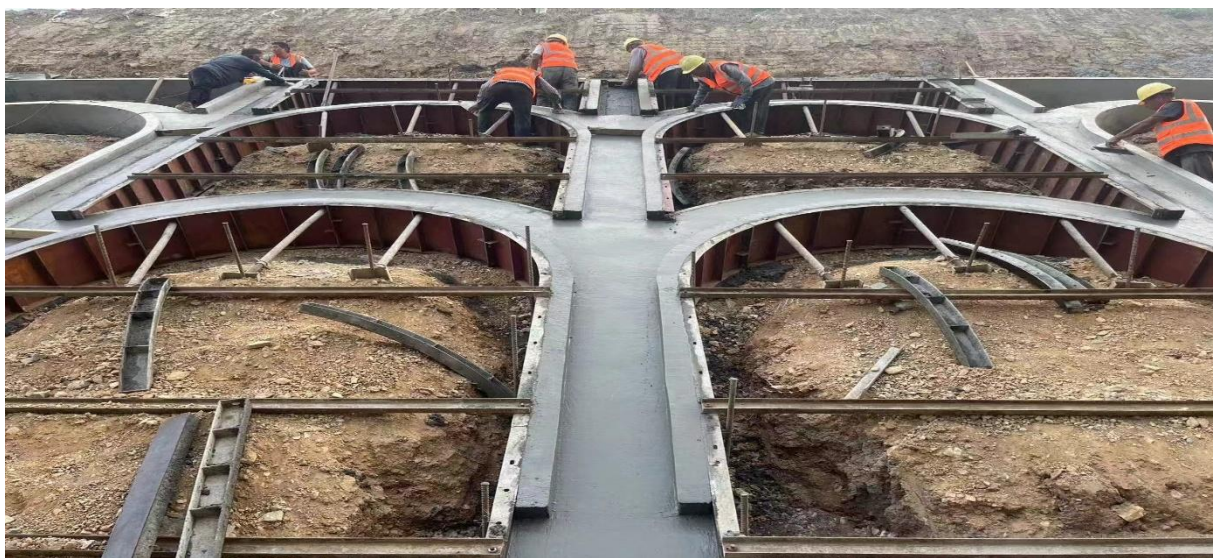
图：阜淮高铁（一分部）路基边坡防护施工现场
